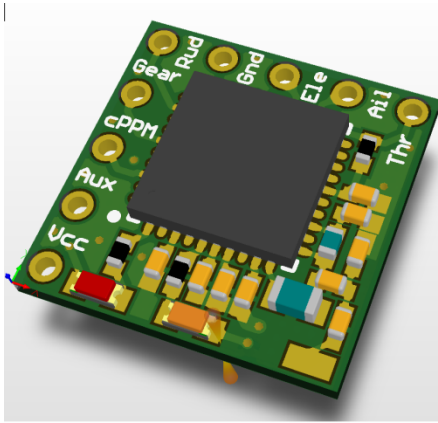
Fig. 1 Top side
